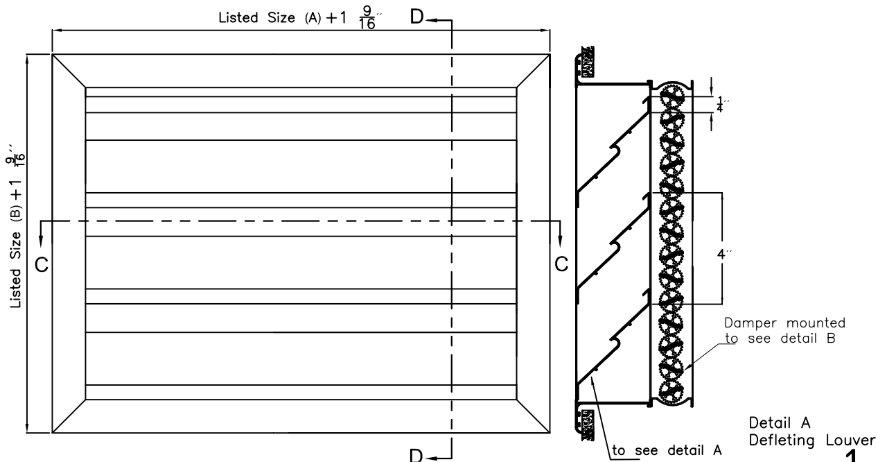
SECTION D-D
